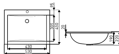
KR 132 BLM
