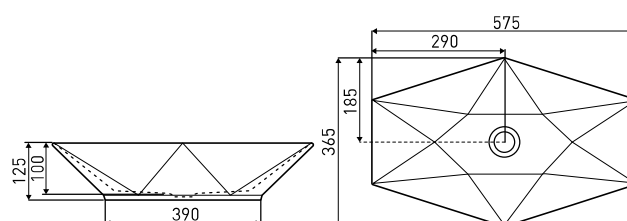
KR 570 BLM
