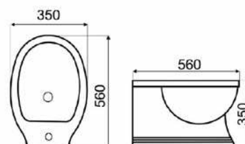
KR 15 RETRO BIDET WISZĄCY
