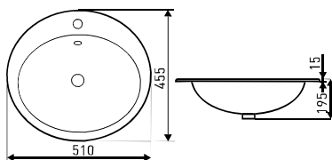
KR 132
