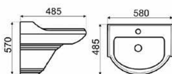
KR 14 RETRO UMYWALKA Z PÓŁPOSTUMENTEM
