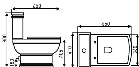
KLEOPATRA 11 KOMPAKT WC
