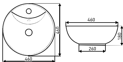
KR 157
